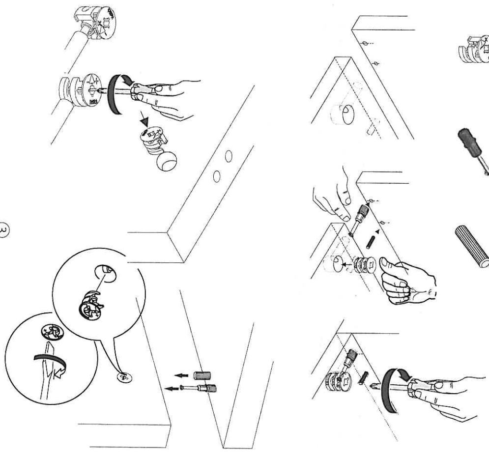
Minifix Körper Minifix Gövde
